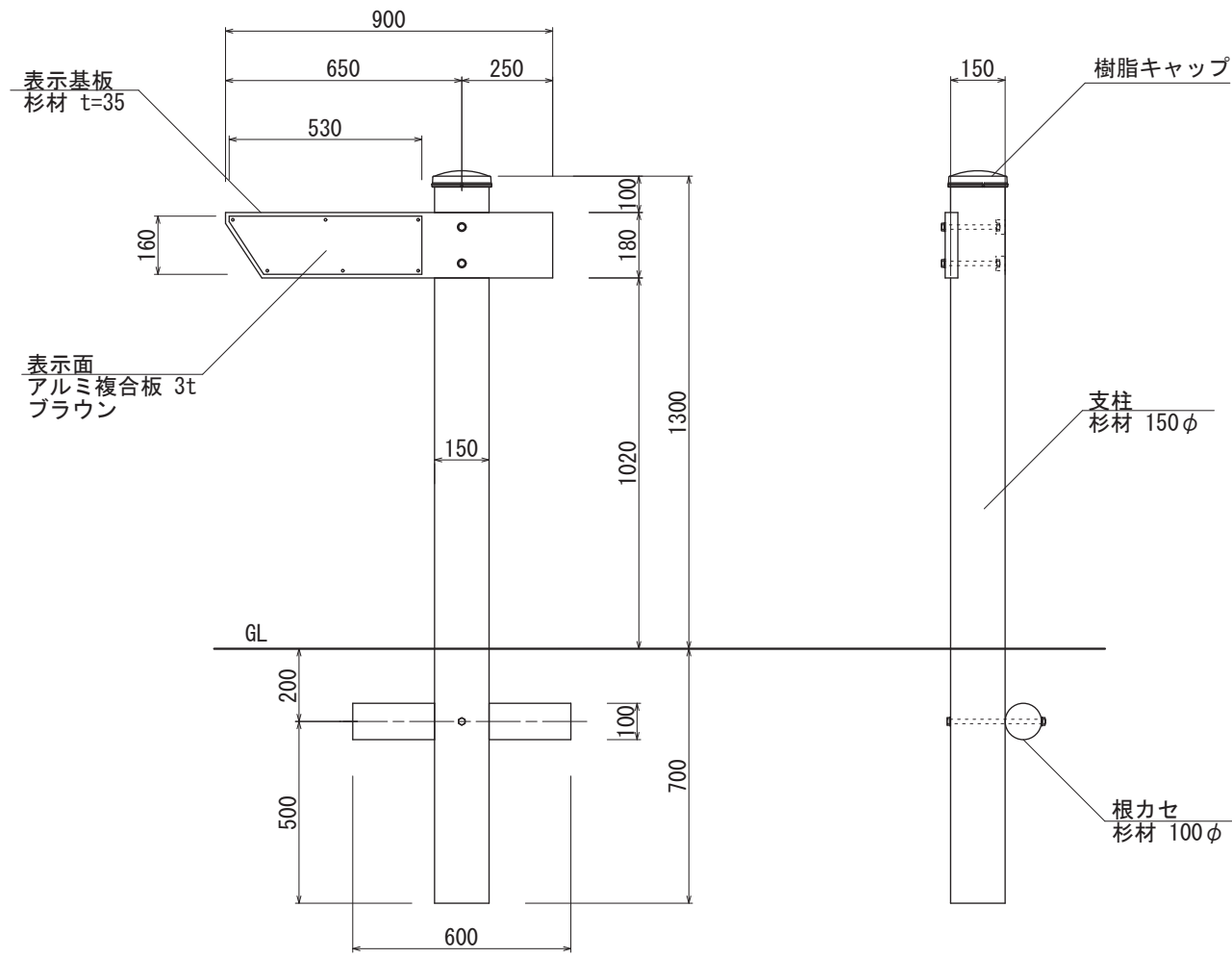
【正面図 S=1:20】
