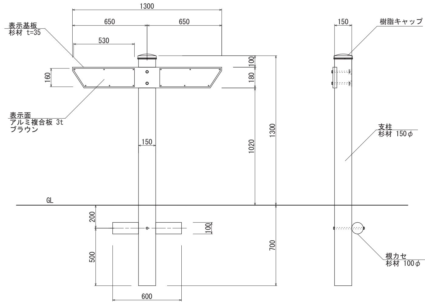
【正面図 S=1:20】
