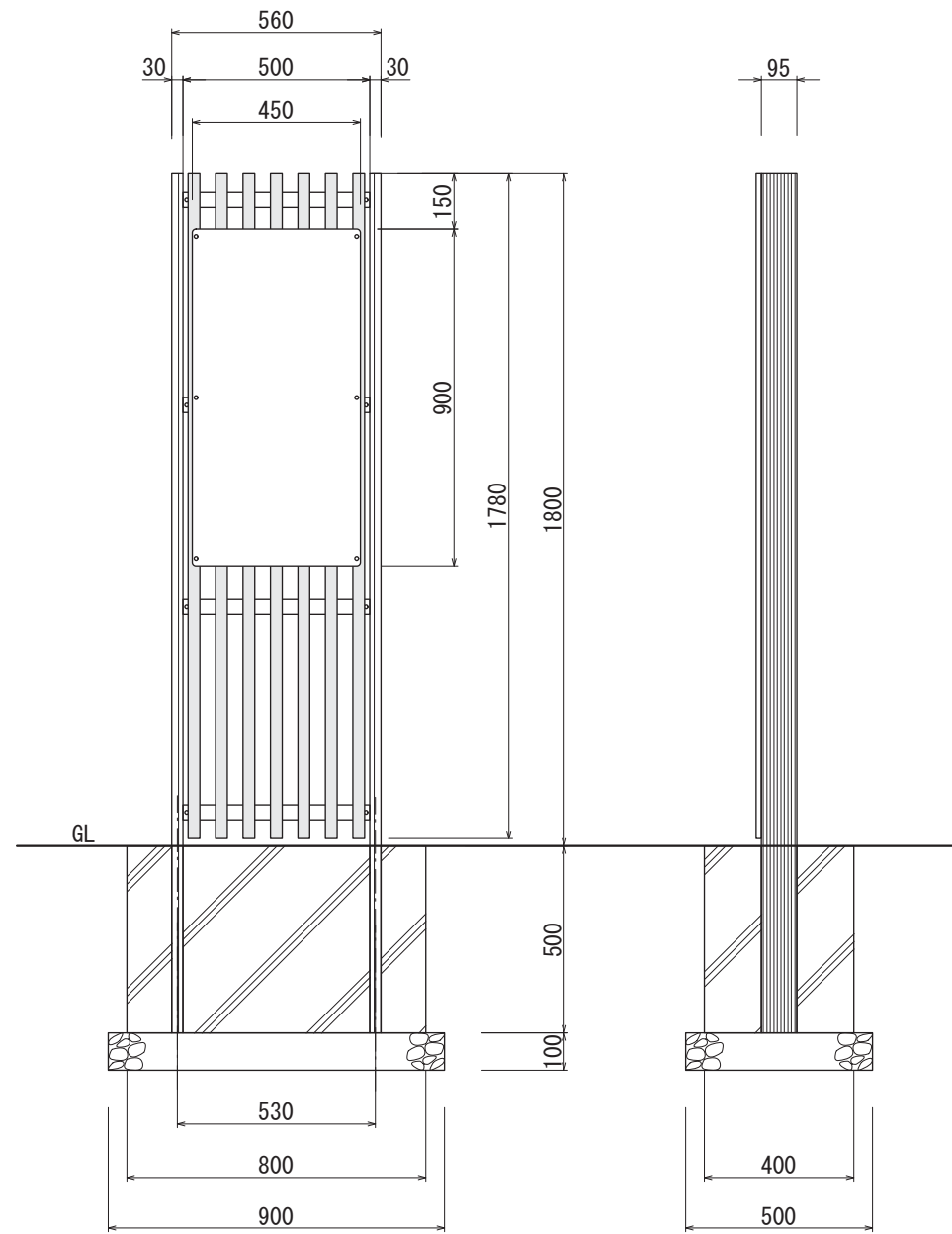
【正面図 S=1:20】
