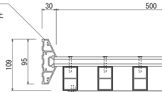
【平面図 S=1:5】
