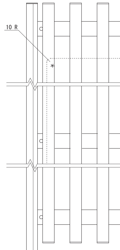
【正面図 S=1:5】
