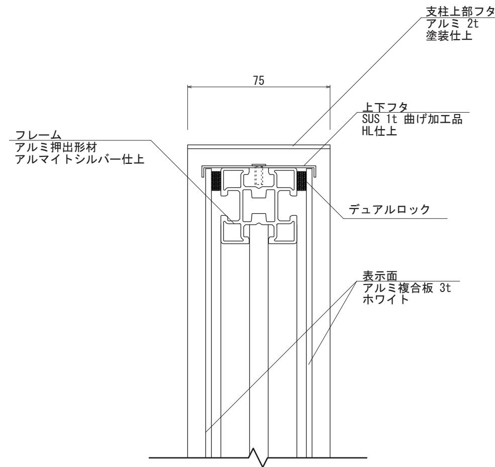
【断面図 S=1:2】
