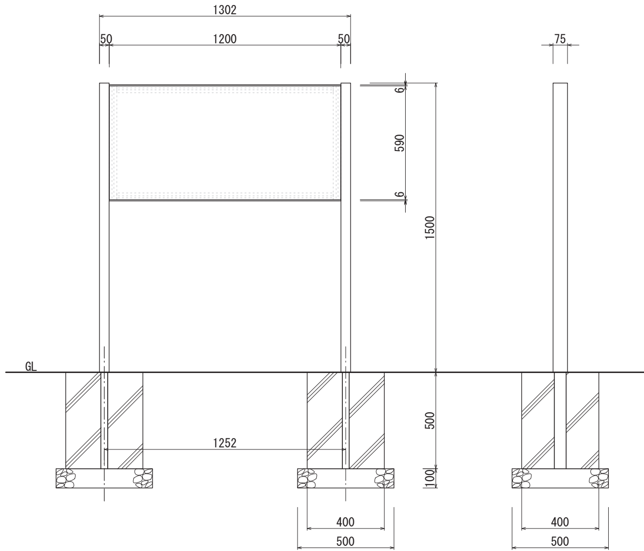
【正面図 S=1:20】
